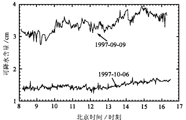
图8 测量的某两天中水汽可降水含量的日变化
