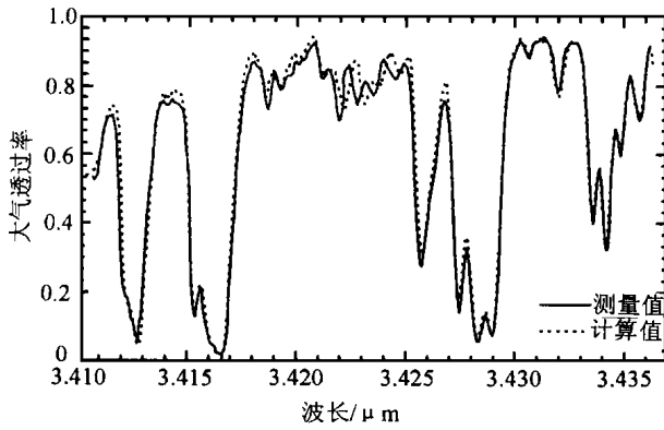
图5 计算和测量的整层大气透过率
