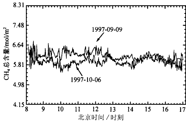
图6 测量的某两天中甲烷总含量的日变化
