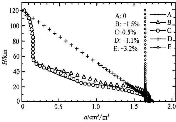
图 2 模式大气中甲烷的混合比廓线
