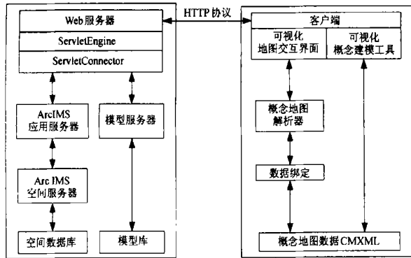
图 2 可视化地学建模环境系统结构图
