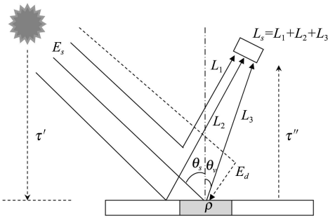
图 1 太阳反射光谱区传感器入瞳处辐射度贡献示意图
