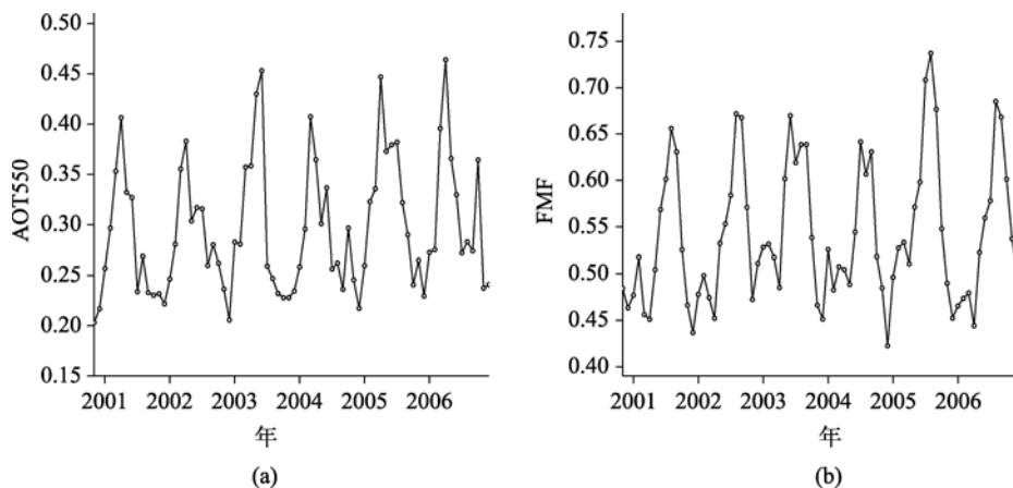
图 5 中国海域区域平均的时间序列 (a) AOT550; (b) FMF
