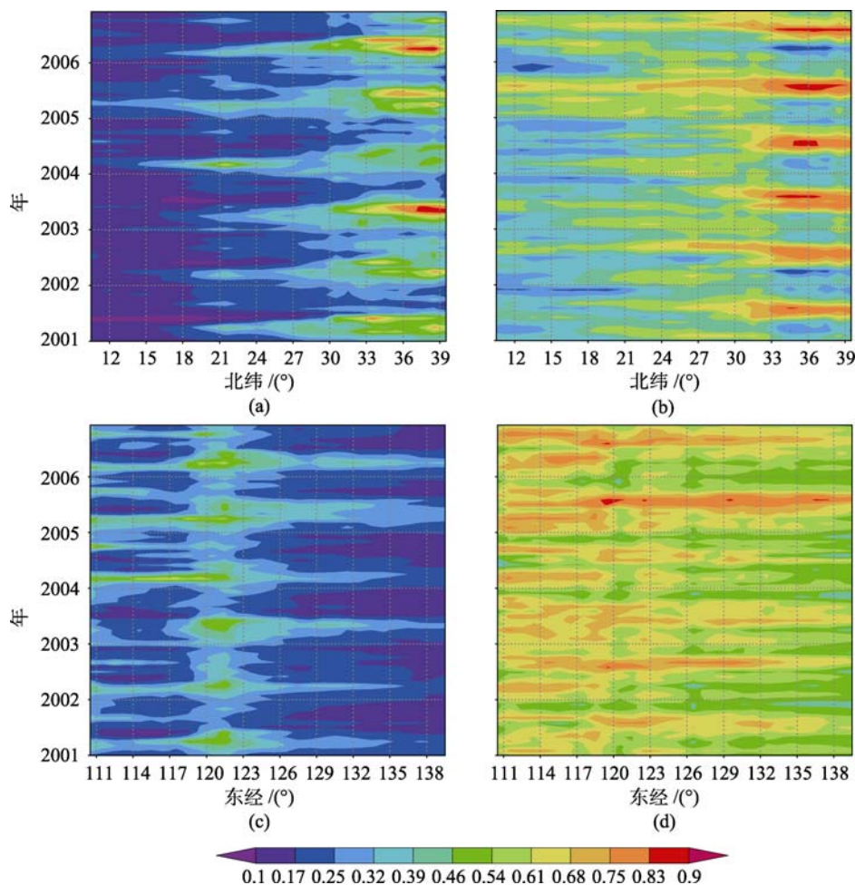
图 7 中国海域 AOT550 和 FMF 的经纬向分布图
