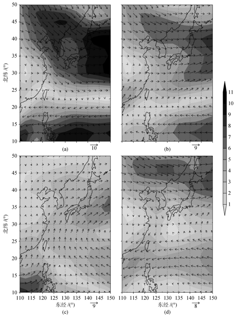
图9 中国海域 2000—2006 年 6a 的 850hp 风场的季节平均 (a) 冬季; (b) 春季; (c) 夏季; (d) 秋季
