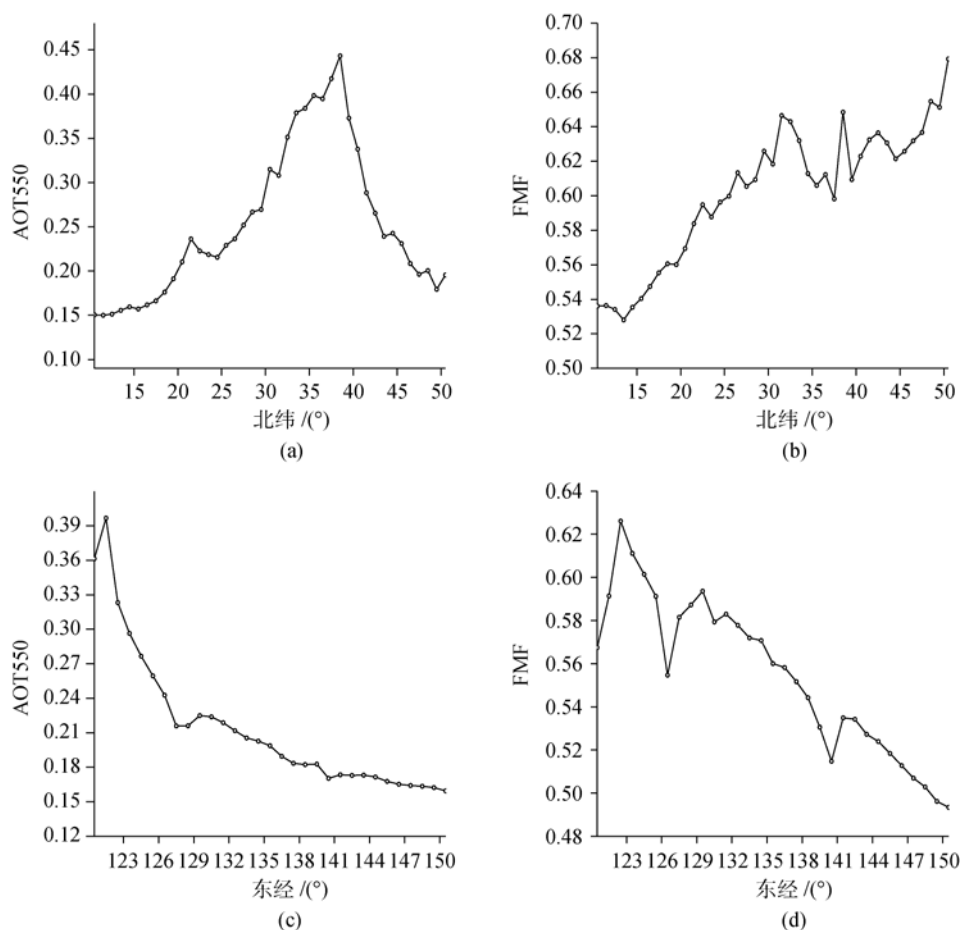
图8 中国海域 6a 区域平均的经纬向变化 (a) 纬向 AOT550; (b) 纬向 FMF; (c) 经向 AOT550; (d) 经向 FMF
