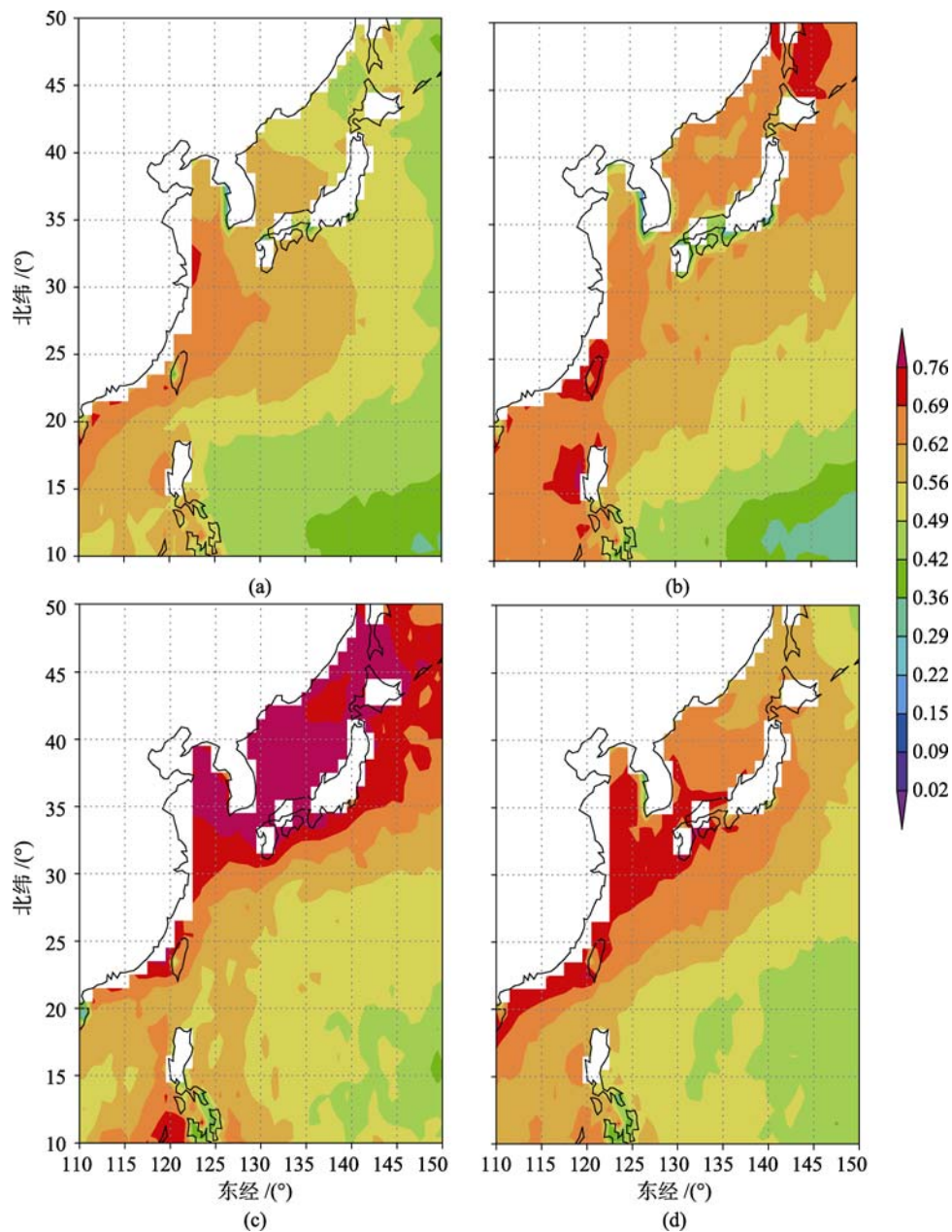
图 4 中国海域小颗粒比例(FMF)的季节分布
