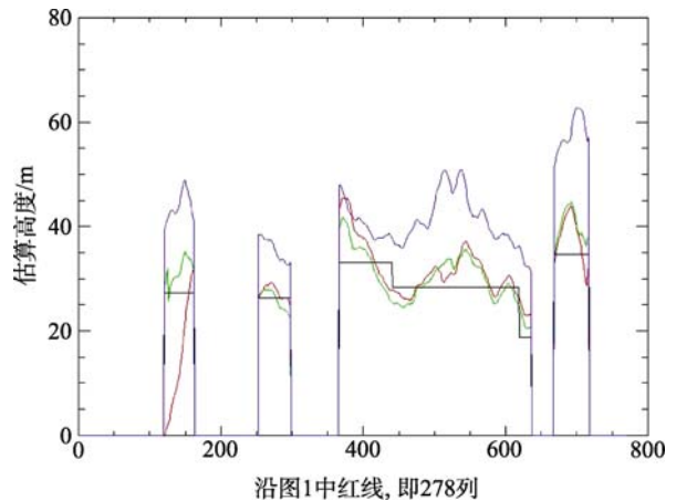
图 10 3 种反演方法估计的平均高的方位向高度剖面图 (紫色: SINC 函数反演法; 红色: 相干相位-幅度综合反演法; 绿色: 改进的相干相位-幅度综合反演法; 黑色: 地面实测平均优势树高)
