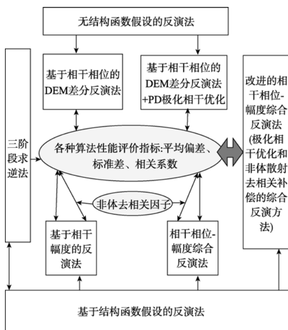
图3 研究技术路线
