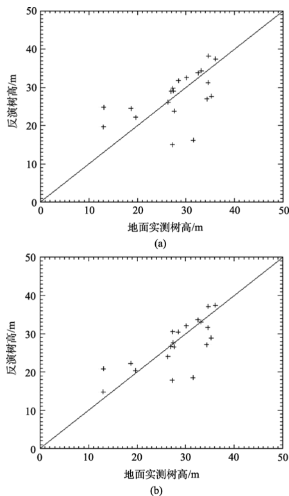
图 8 基于相干相位-幅度综合反演法求算的平均树高和地面实测平均树高的散点图
