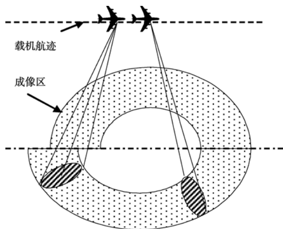
图 1 环视模式示意图
