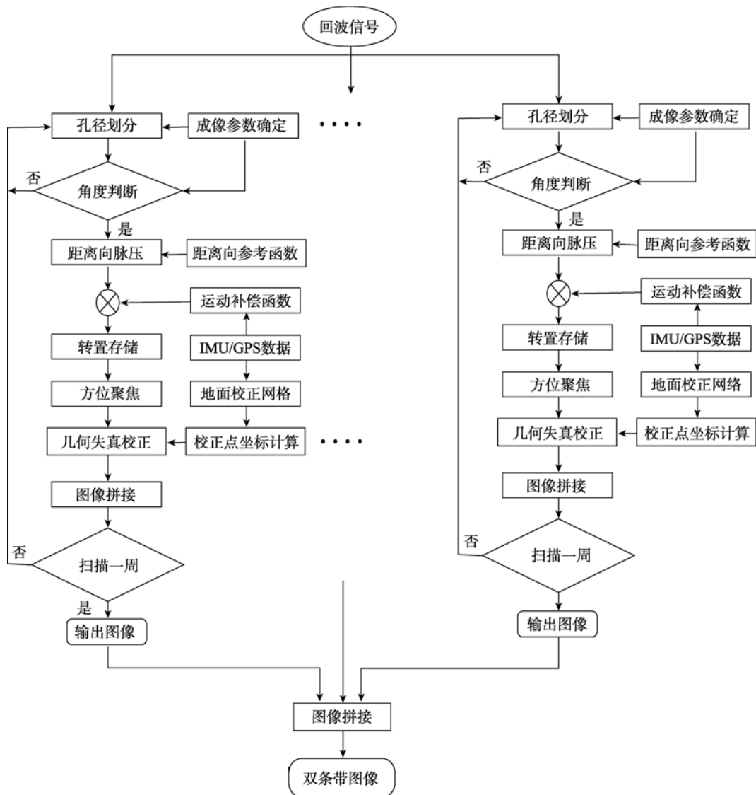
图 6 双条带 SAR 信号处理流程图
