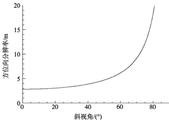
图 7 方位向分辨率与斜视角关系曲线
