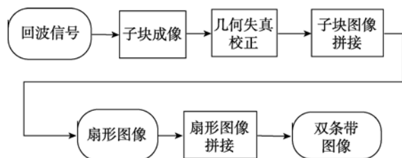
图3 双条带 SAR 成像处理框图
