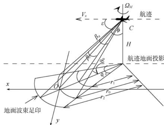
图4 环视 SAR 系统成像的几何关系
