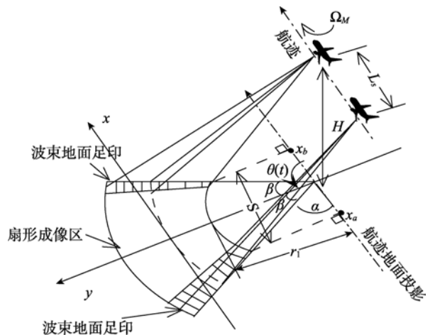
图 8 双条带 SAR 无缝拼接条件示意图
