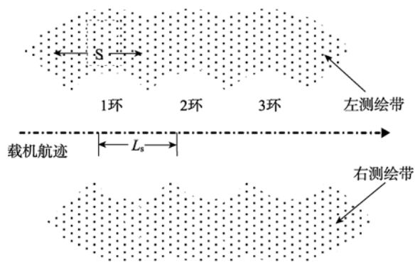
图2 双条带 SAR 工作模式示意图
