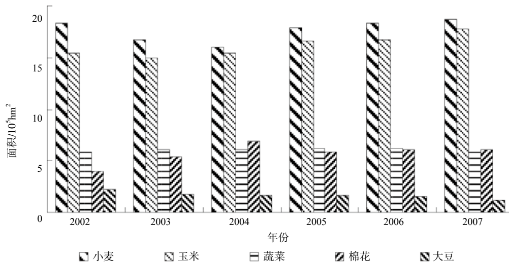
图6 2002年—2007年作物种植面积图
