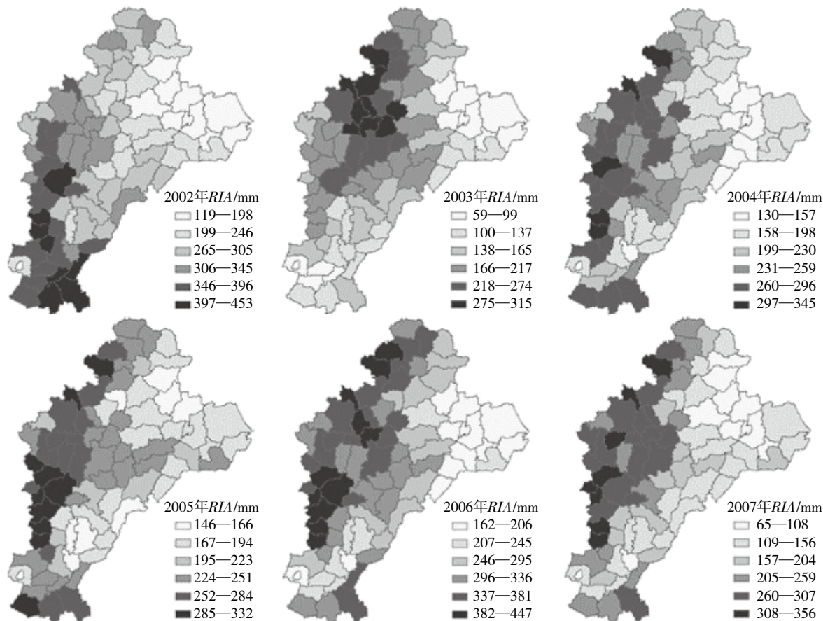
图2 2002年—2007年灌溉需水量的空间分布
