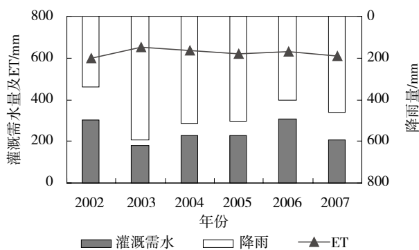
图3 不同年份年均灌溉需水量、降雨量和蒸散发量的比较(2002年—2007年)
