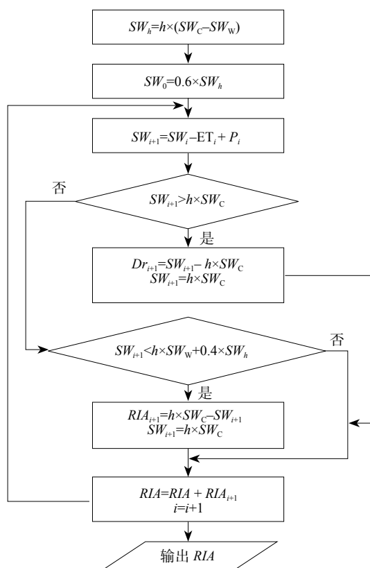
图1 灌溉需水量计算流程图
