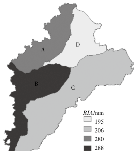
图4 各流域年平均灌溉需水量(A、B、C、D分别代表大清河淀西平原、子牙河平原、黑龙港及运东平原和大清河淀东平原)
