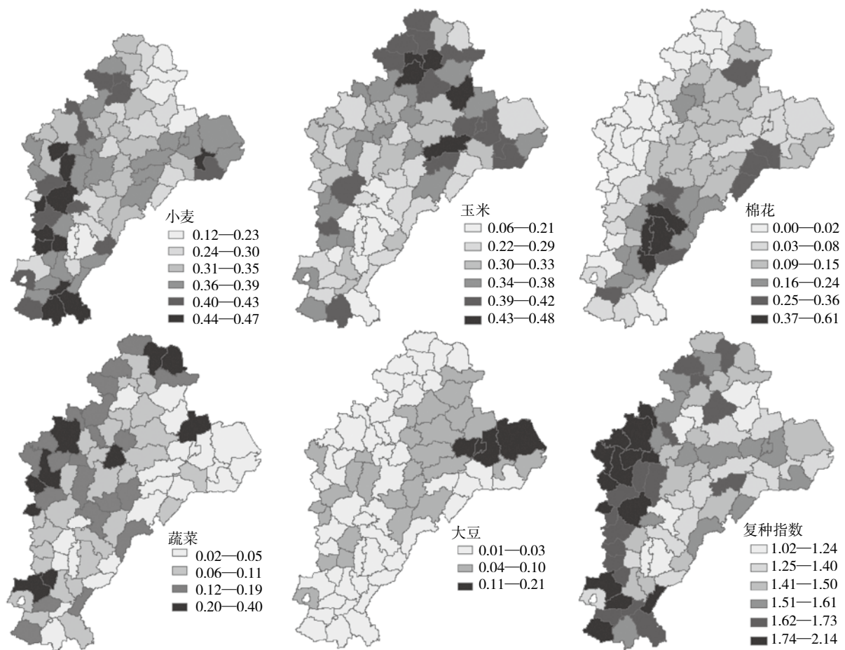
图7 各县作物种植面积占总种植面积的比例及复种指数分布图(2002年—2007年)
