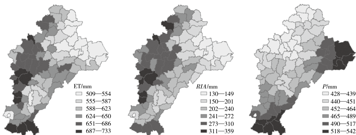
图5 多年平均蒸散发量(ET), 灌溉需水量(RIA)和降雨量(P)
