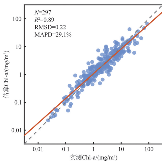
(a) MLP-NN 反演结果与实测值对比散点图
