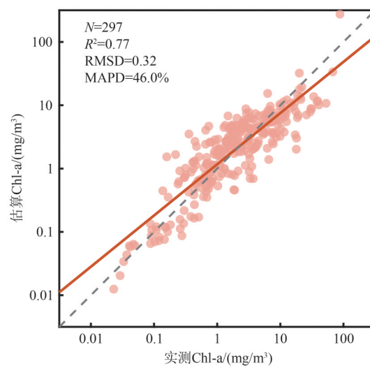
(b) OCI 反演结果与实测值对比散点图
