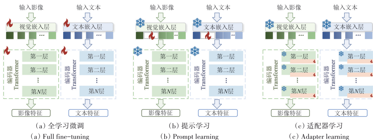
图5 基于跨模态预训练模型的3种微调策略示意图
