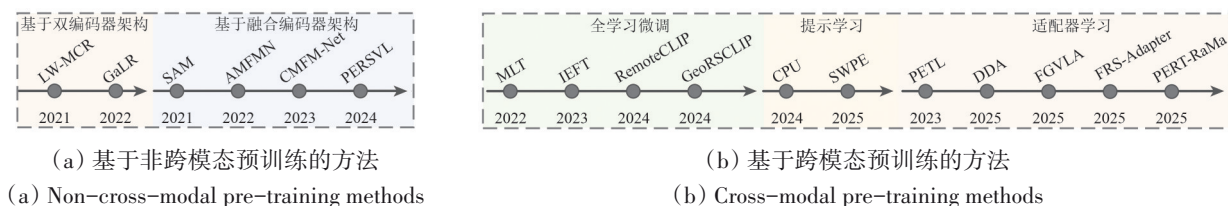
图4 RS-CMITR任务方法演进时间轴
