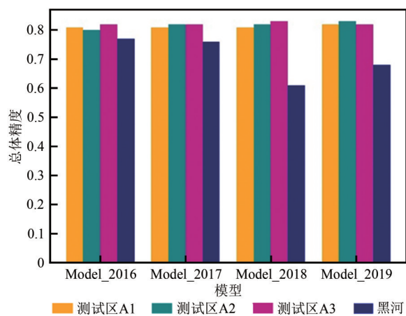
图7 不同模型在测试区预测当年数据的总体精度
