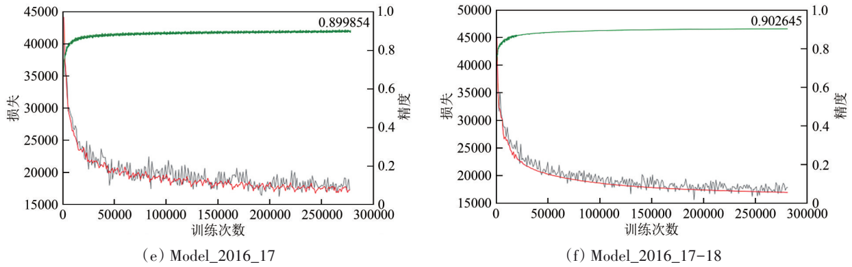
图4 模型训练 Loss 图
