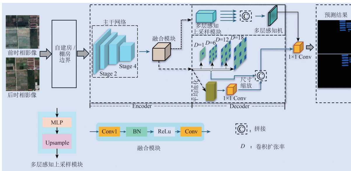
图1 DHRformer网络结构图
