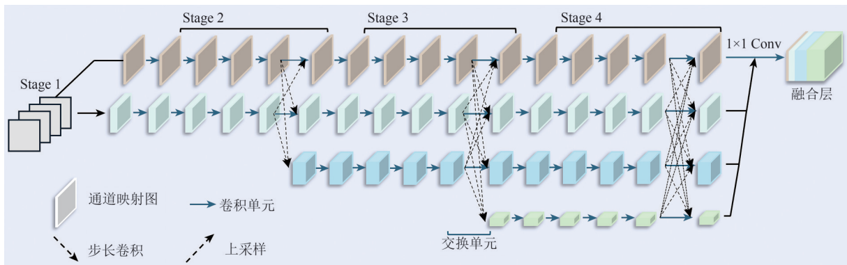
图2 HRNet 高分辨率网络结构
